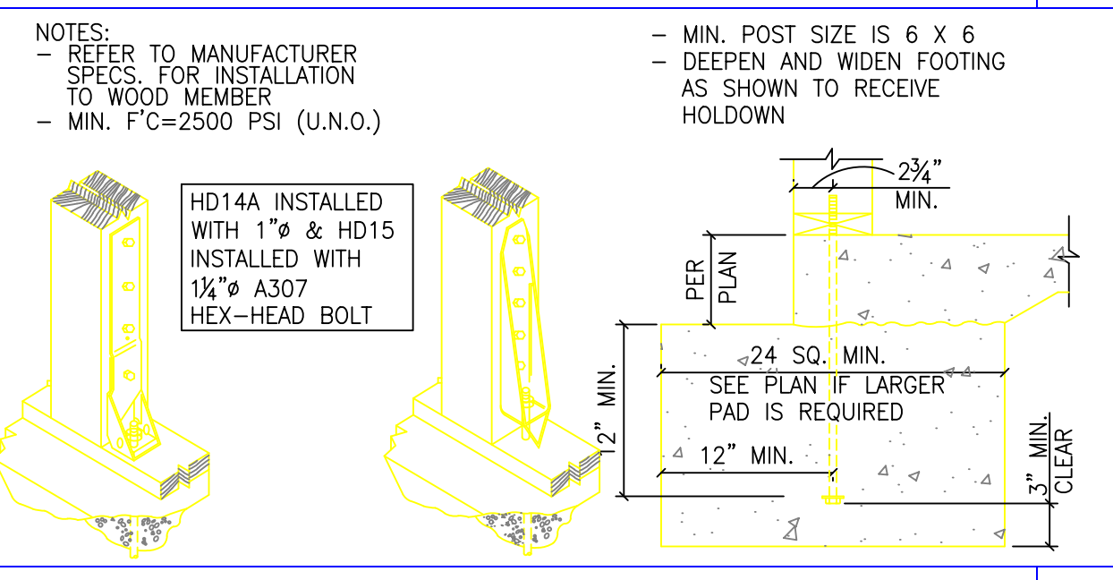
HD14A/HD15 HOLDOWN INST. 17
